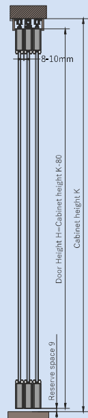
2+1 Door
