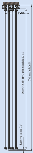
3+1 Door
